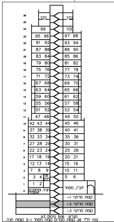
חתך טכני:
